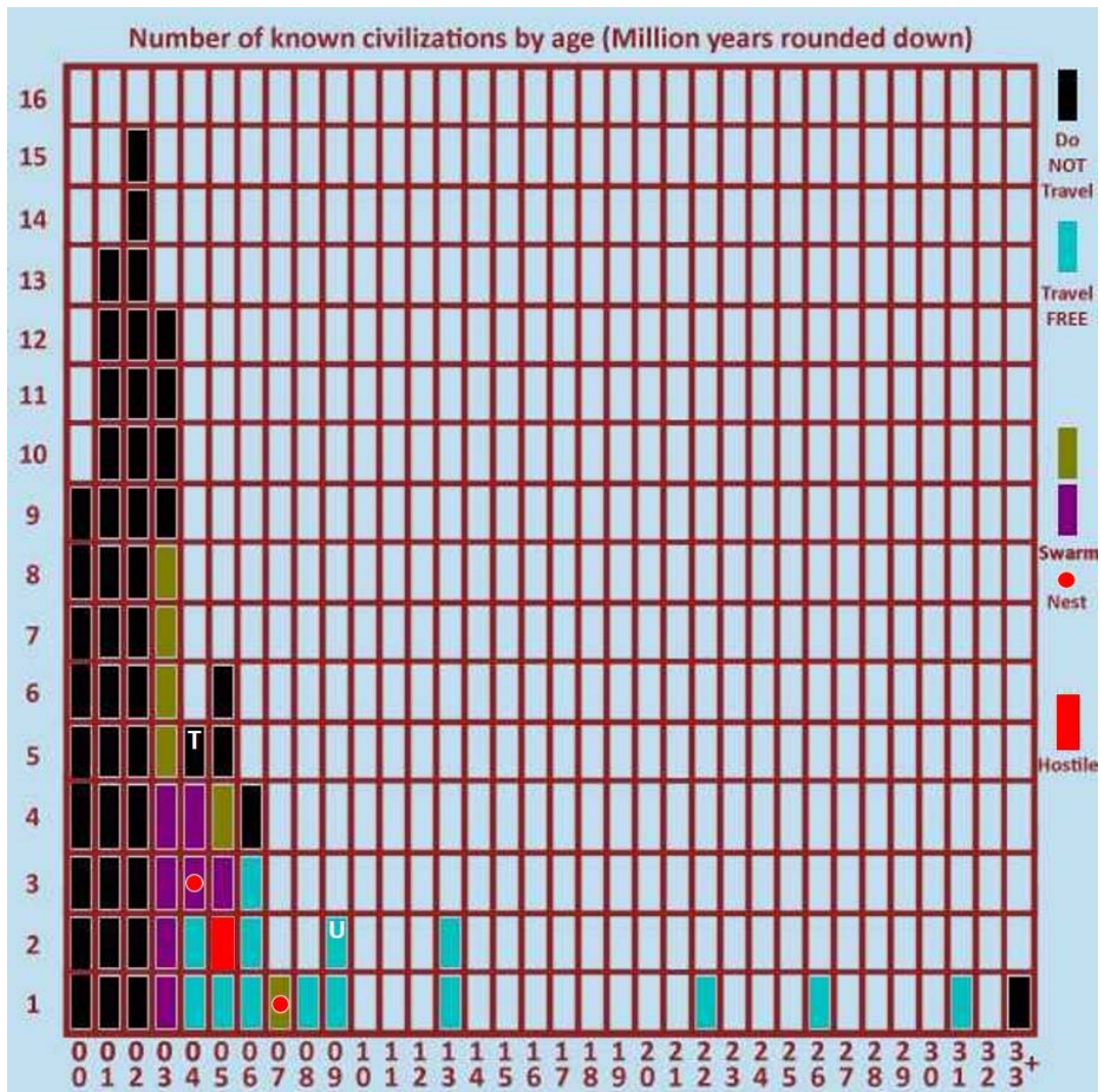
Civilizaciones planetarias identificadas por U. Explicación en el texto.
